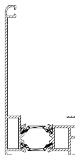
Spodní AL profil jednoduchý s přerušným tepelným mostem
